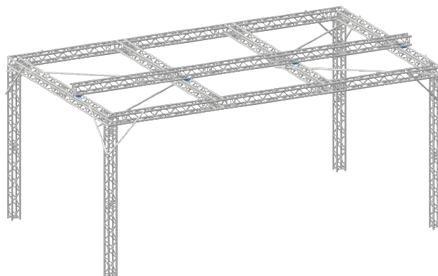
1 Truss System Hoop Scale: 1:50
